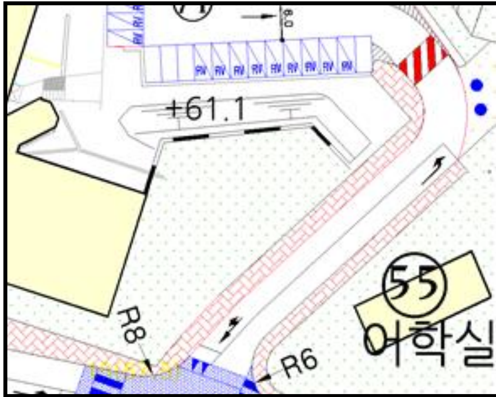
경상대 측면 주차장 개설신규개설 도면
